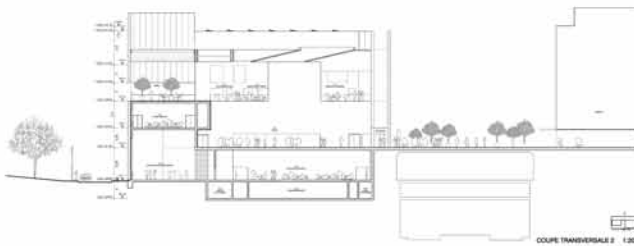
COUPE TRANSVERSALE 1 1:200
