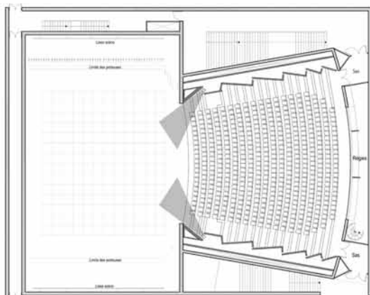
Plan de la salle frontale 565 places Ech. 1/100 e
