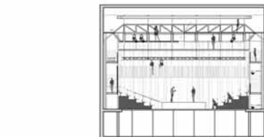
Coupe transversale de la salle modulable Ech. 1/100 e
