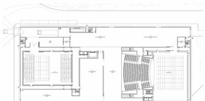
PLAN NIVEAU -1 1/200
