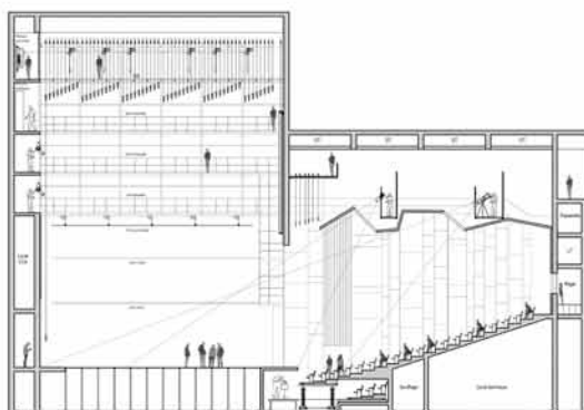
Coupe longitudinale de la salle frontale Ech. 1/100 e
