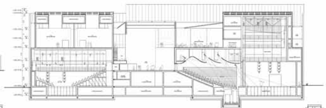
COUPE LONGITUDINALE AX 1/200
